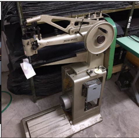
#14 Machine à coudre de cordonnier Metro Spezial.
